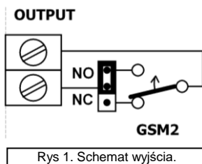
Rys 1. Schemat wyjścia.
